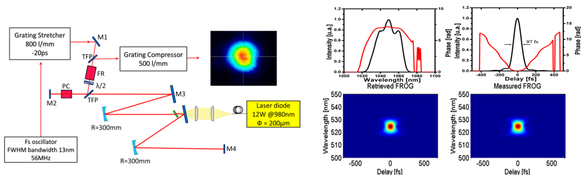
Fig. 1.(gauche) Dispositif expérimental et profil du faisceau amplifié. M : miroir plan . TFP : polariseur à film mince. PC: Cellule de pockels. FR: Rotateur de Faraday. (droite) (haut) Profils spectraux et temporels retrouvés à partir du FROG SHG ; (bas) traces FROG mesurées et retrouvées.
