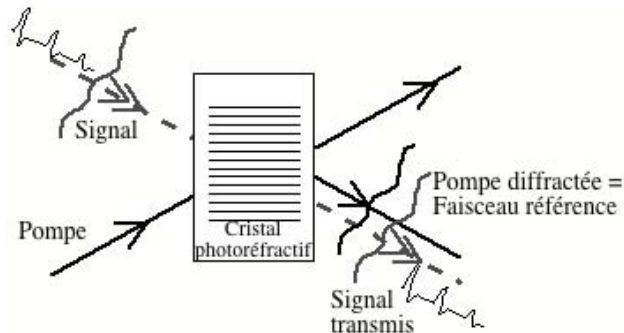
Figure 2. Principe de fonctionnement du capteur optique d'ultrasons par mélange à deux ondes dans un cristal photoréfractif.
